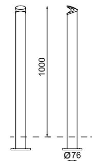
SBD100 столбик оградительный
