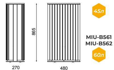
MIU511 / MIU512 урна для мусора
