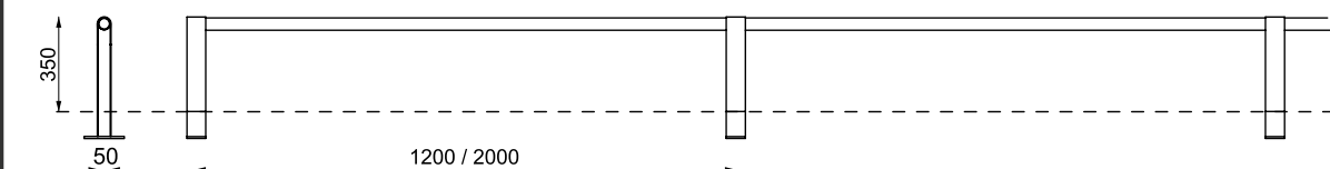
SC500 ограждение низкое
