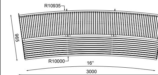
LDP151-a5 Высокая скамья изогнутая
