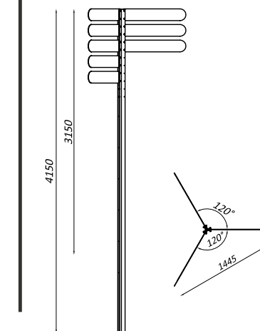
NUK130 указатель направлений
