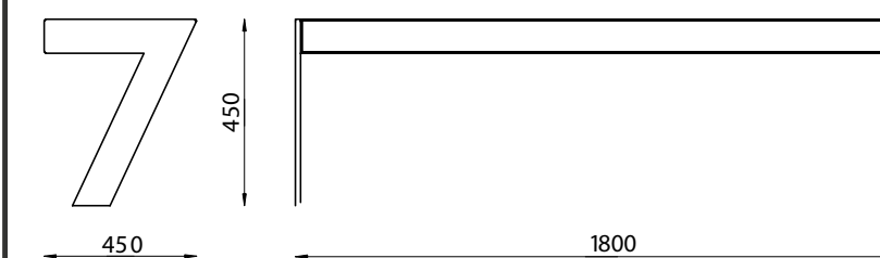
PZ 02 / PZ 02-01 скамья
