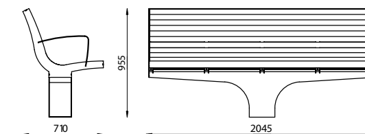
GR S20 B скамья со спинкой
