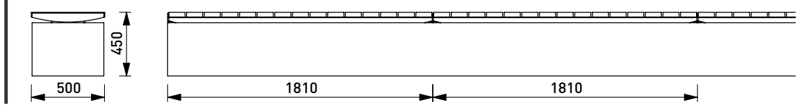
LVS30 / LVZ60 / LVZ61 модульный комплект парковой скамейки
