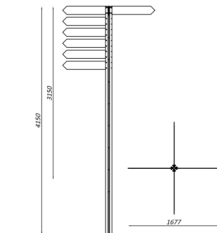
NUK140 указатель направлений
