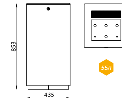
Polygood Cube A PG321 / с пепельницей
