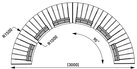
LVS31-e / LVS60 / LVS61 / LVS62 комплект изогнутых скамей со спинкой
