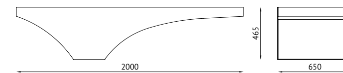
GR S50 скамья без спинки и подлокотников
