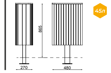
MIU110 / MIU-B110 урна для мусора на центральной опоре
