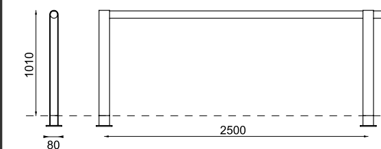
SC600 ограждение с трубкой
