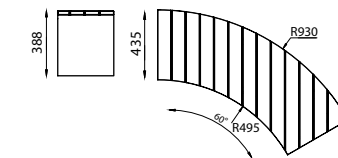
IR495 скамья радиусная
