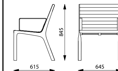
VLA157 скамья с опорной спинкой и подлокотниками
