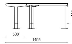
LVS510 изогнутая скамья
