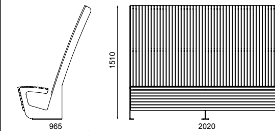
LDP150 Высокая скамья
