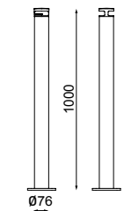
DON100 столбик оградительный
