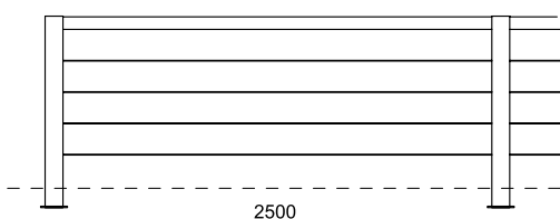
SC700 ограждение с тросом из нержавеющей стали
