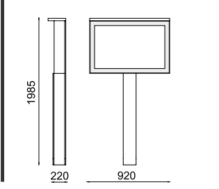
IF220 односторонняя информационная витрина (900 x 700 мм)
