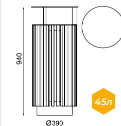
DG115 урна с крышкой
