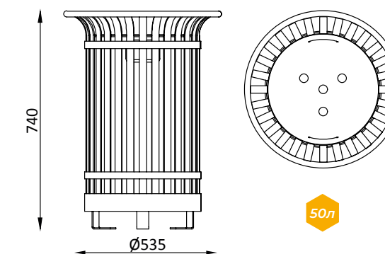
CLASSIC 50 CLS150 урна для мусора
