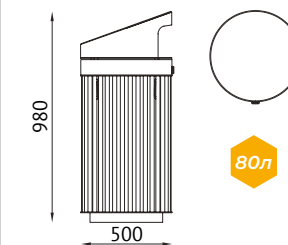
GR LB120 урна для мусора
