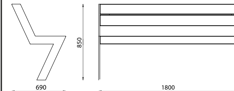
PZ 01 / PZ 01-01 скамья
