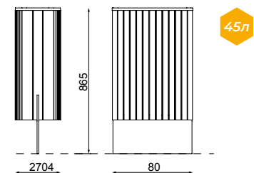
MIU410 / MIU-B410 урна для мусора на стальной плите
