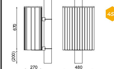
MIU010 / MIU-B010 урна для мусора с боковым креплением
