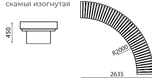
BANK RING 90R2000 BNK412 скамья изогнутая
