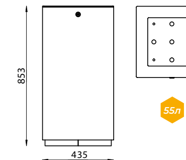
Polygood Cube PG320 урна для мусора
