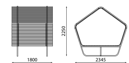
SHELTER RELAX ILU350 НАВЕС-СКАМЬЯ
