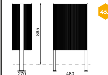
MIU200 / MIU-B200 урна для мусора на двух опорах
