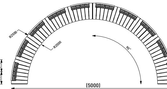
LVS32-a / LVZ60 / LVZ61 комплект изогнутых скамей со спинкой
