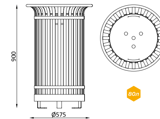
CLASSIC 80 CLS180 урна для мусора
