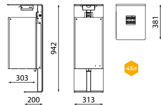
PURE урна для мусора
