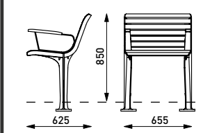
EMS357 скамья с опорной спинкой и подлокотниками
