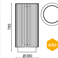
DG110 урна для мусора
