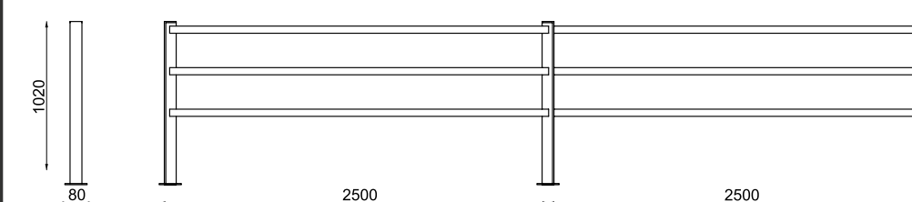
SL730 ограждение с трубками
