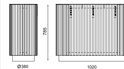
DG610 урна тройная
