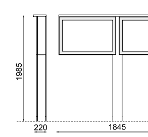
IF220 односторонняя информационная витрина (900 x 700 мм)
