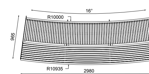
LDP151-e5r Высокая скамья изогнутая
