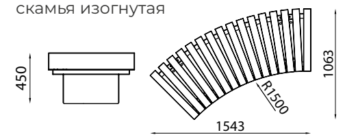
BANK RING 45R1500 BNK310 скамья изогнутая
