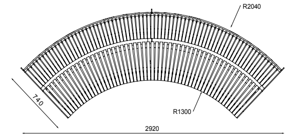
LPC150-a скамья изогнутая
