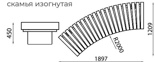
BANK RING 45R2000 BNK410 скамья изогнутая
