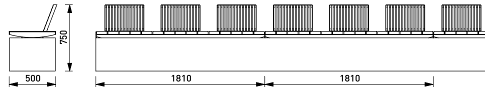
LVS70 / LVZ60 / LVZ61 комплект скамей со спинкой
