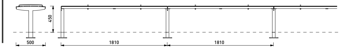
LVS15 / LVS50 / LVS51 комплект удлиненной скамьи на центральной ножке
