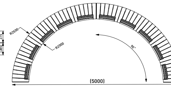
LVS32-e / LVZ60 / LVS61 комплект изогнутых скамей со спинкой
